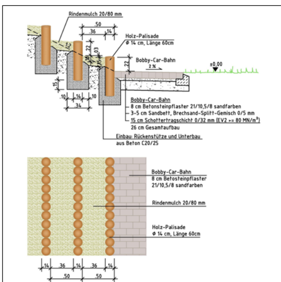
Detail: Ausgang Kletterhügel
