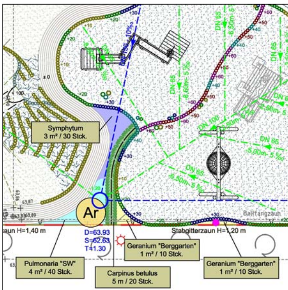
Detail: Sandspielbereich am Gebäude
