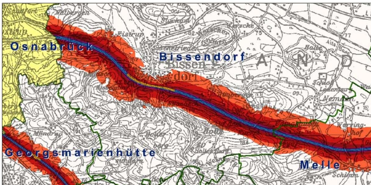
Isophonenplan
