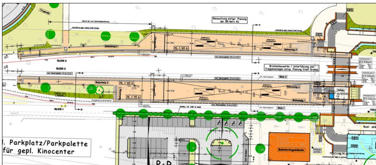
Auszug aus Gesamtlageplan
