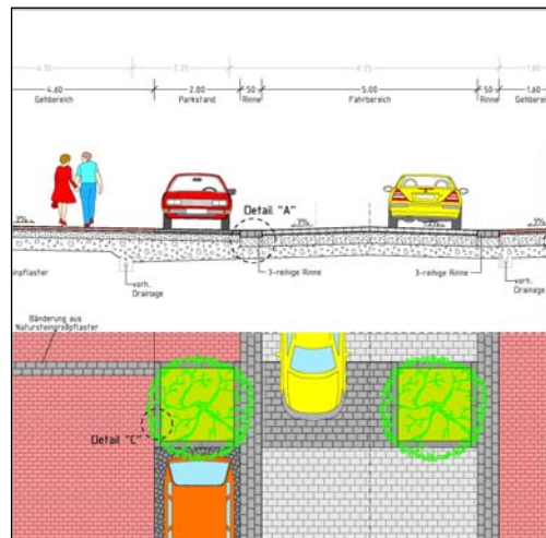
Querschnitt mit Draufsicht
