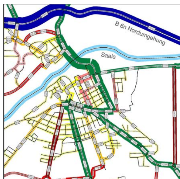
Netzbelastungsplan Prognose 2015
