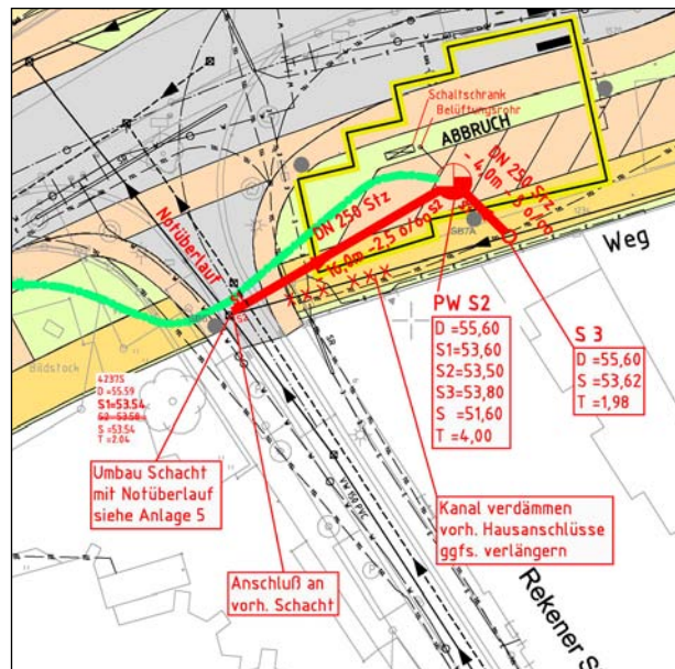
Neubau SW-Pumpwerk als Maßnahme des ABK
