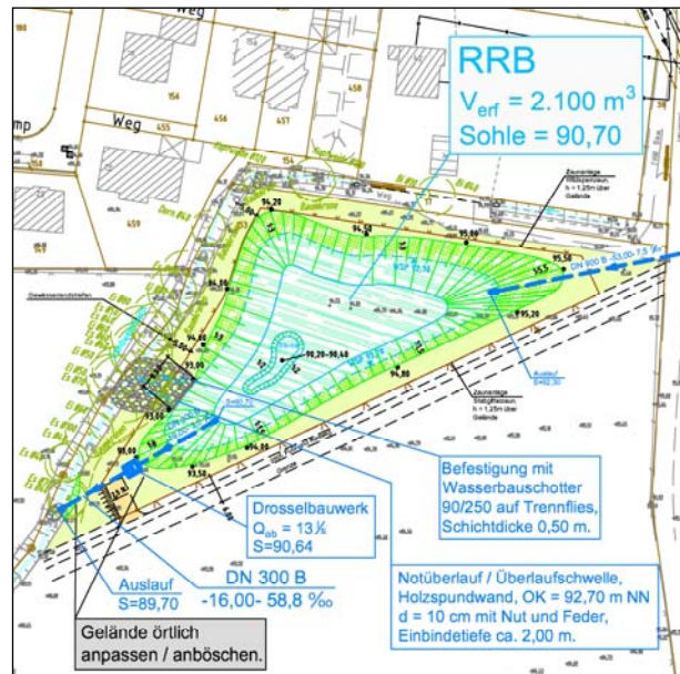
Regenrückhaltebecken
